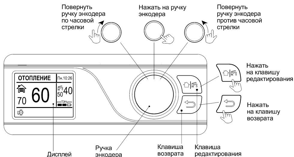
Рисунок 1. Элементы блока управления
