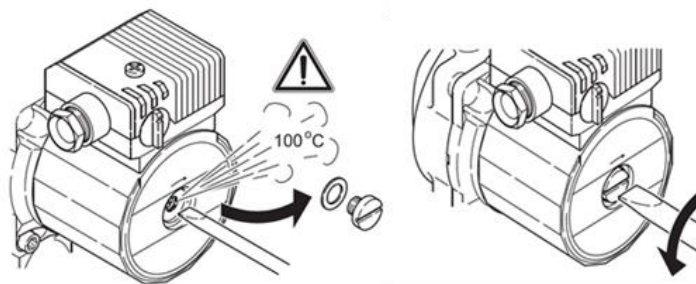
Поворот вала насоса
