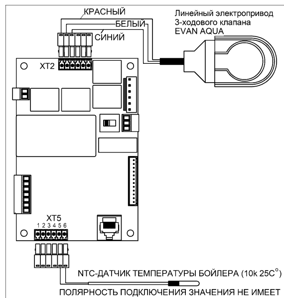
Рисунок 28. Схема подключения 3-ходового клапана ГВС совместно с НТС-датчиком
