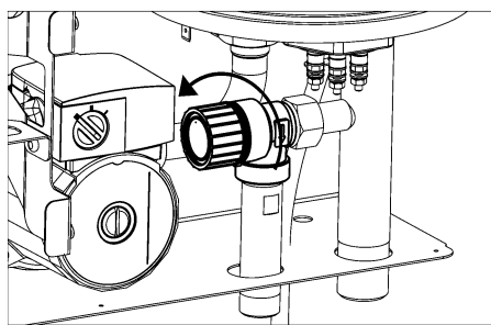
Рисунок 35. Поворот крышки клапана
