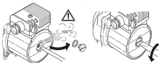
Рисунок 34. Проверка вала насоса
