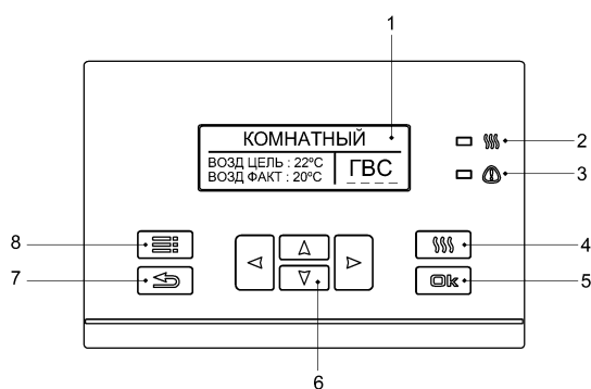
Рисунок 2. Блок управления
