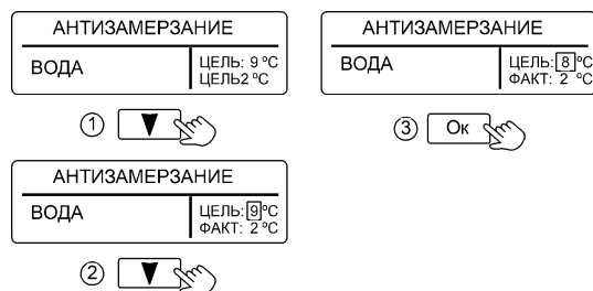
Рисунок 6. Настройка режима «АНТИЗАМЕРЗАНИЕ»
