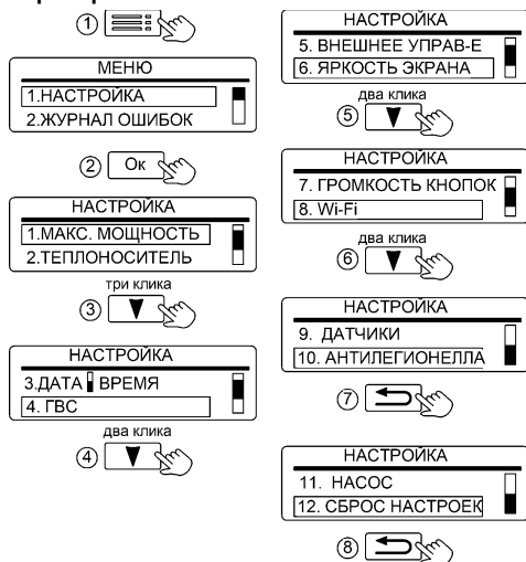
Рисунок 15. Вид вкладки настройка
