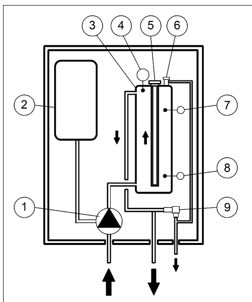
Рисунок 1. Принципиальная схема котла
