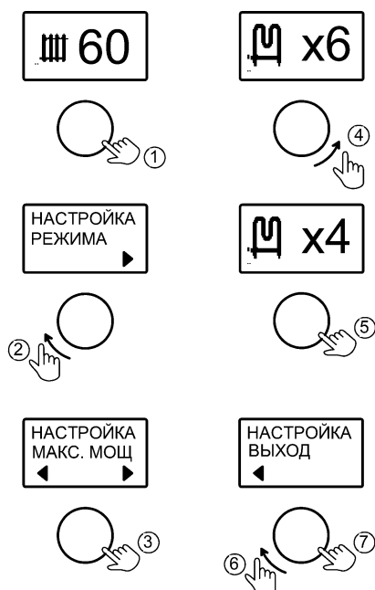
Рисунок 8. Настройка мощности котла
