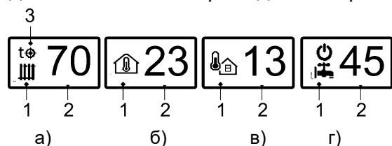
Рисунок 3. Виды главного окна а) режим «ОТОПЛЕНИЕ»; б) режим «КОМНАТНЫЙ»; в) режим «УЛИЧНЫЙ» г) режим «ГВС».
