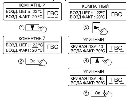
Рисунок 10. Настройка ограничения температуры и кривой ПЗУ
