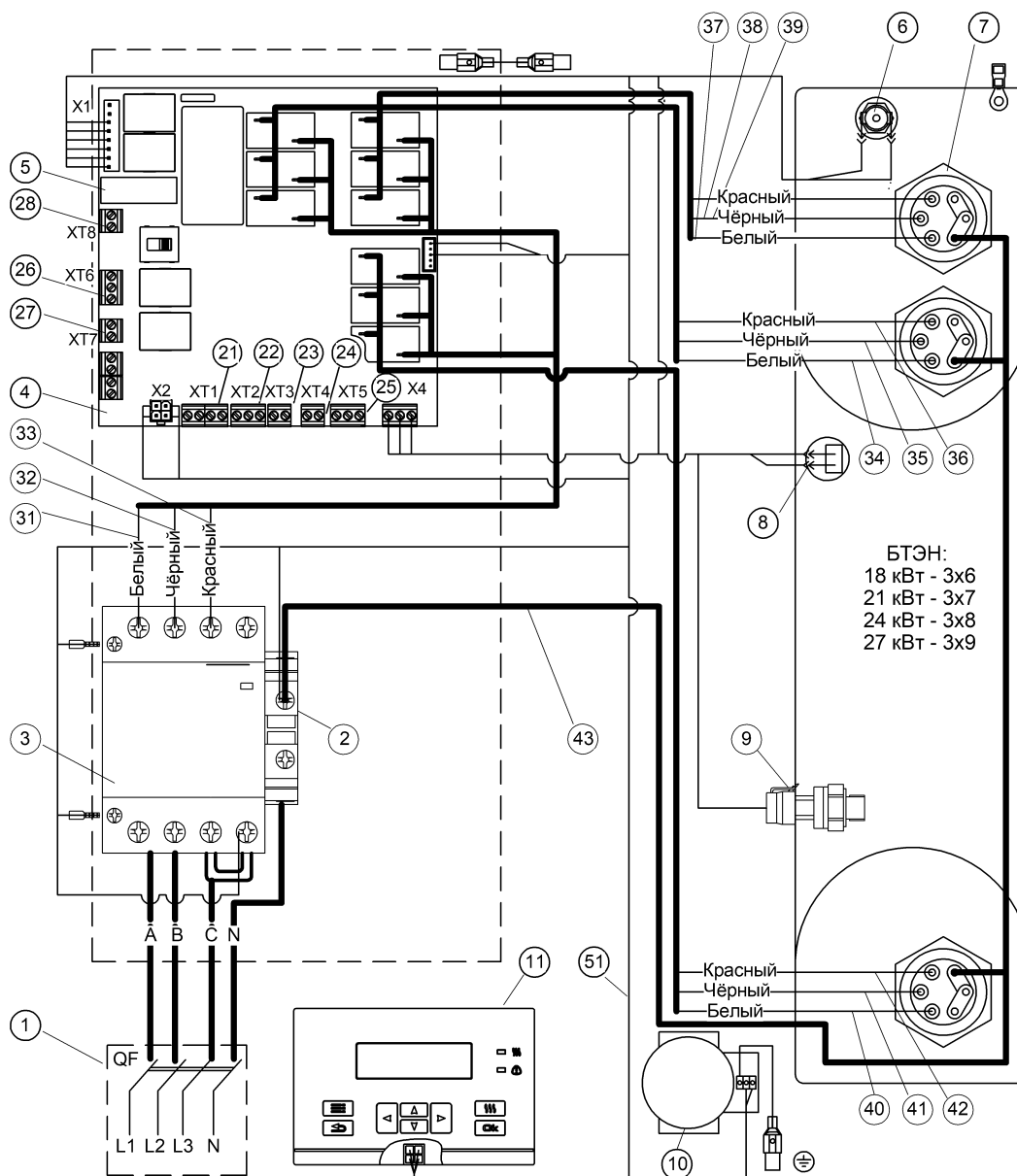
Рисунок 26. Электромонтажная схема EVAN EXPERT PLUS -18...27
