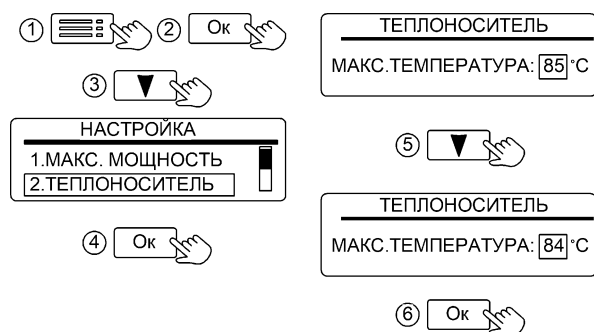
Рисунок 17. Настройка ограничения максимальной температуры теплоносителя
