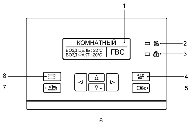
Рисунок 2. Блок управления
