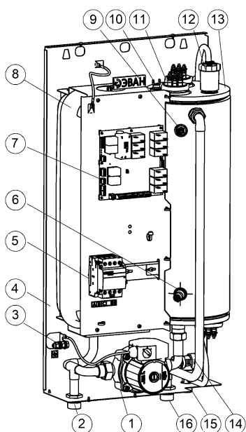
Рисунок 2. Общий вид прибора
