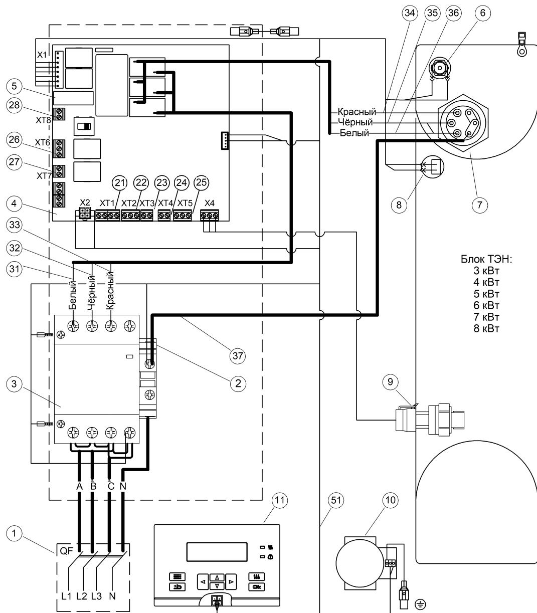
Рисунок 24. Электромонтажная схема подключения EVAN EXPERT PLUS -3...8 к сети 380 В
