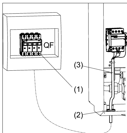
Рисунок 7. Подключение прибора к электросети
