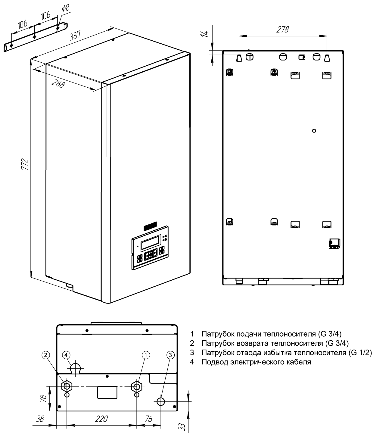
Рисунок 19. Габаритные и присоединительные размеры прибора
