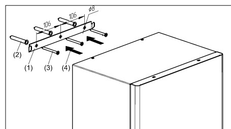
Рисунок 4. Установка прибора на вертикальное основание
