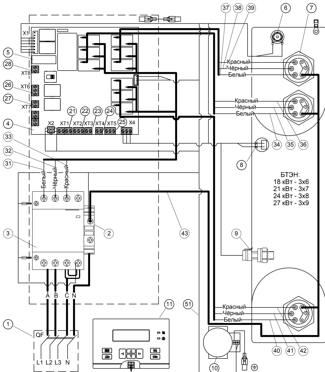
Рисунок 26. Электромонтажная схема EVAN EXPERT PLUS -18...27
