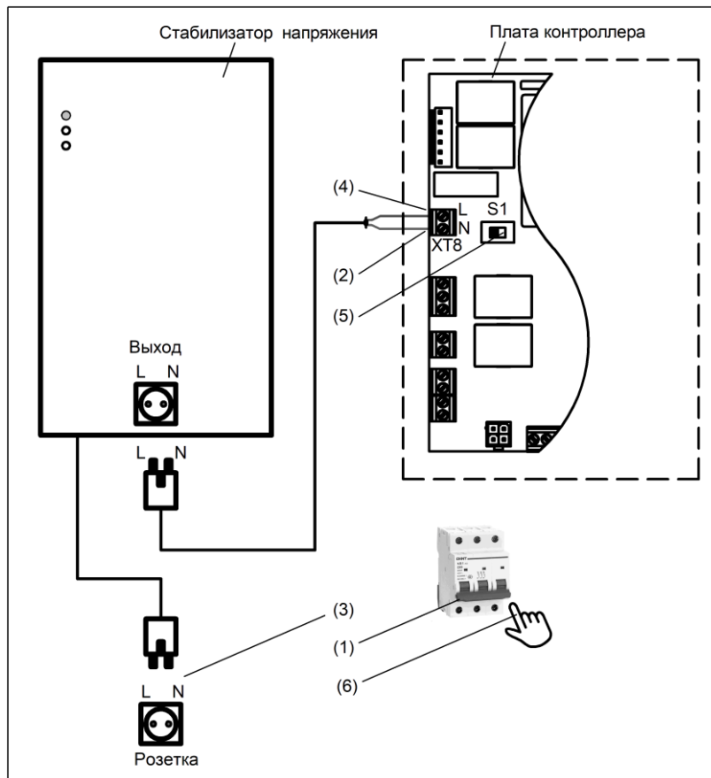
Рисунок 27. Схема подключения стабилизатора напряжения
